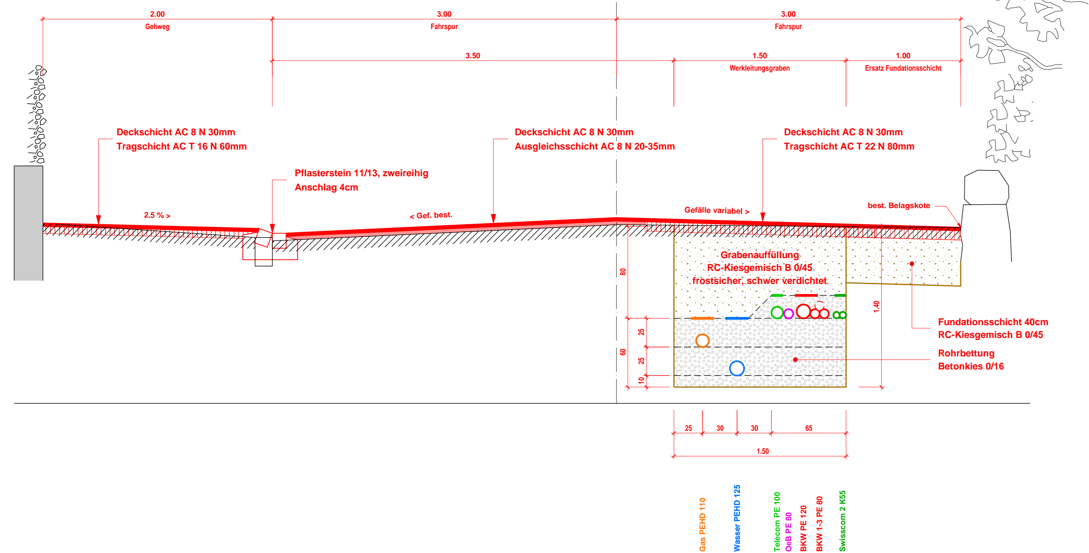
Normalprofil 1
