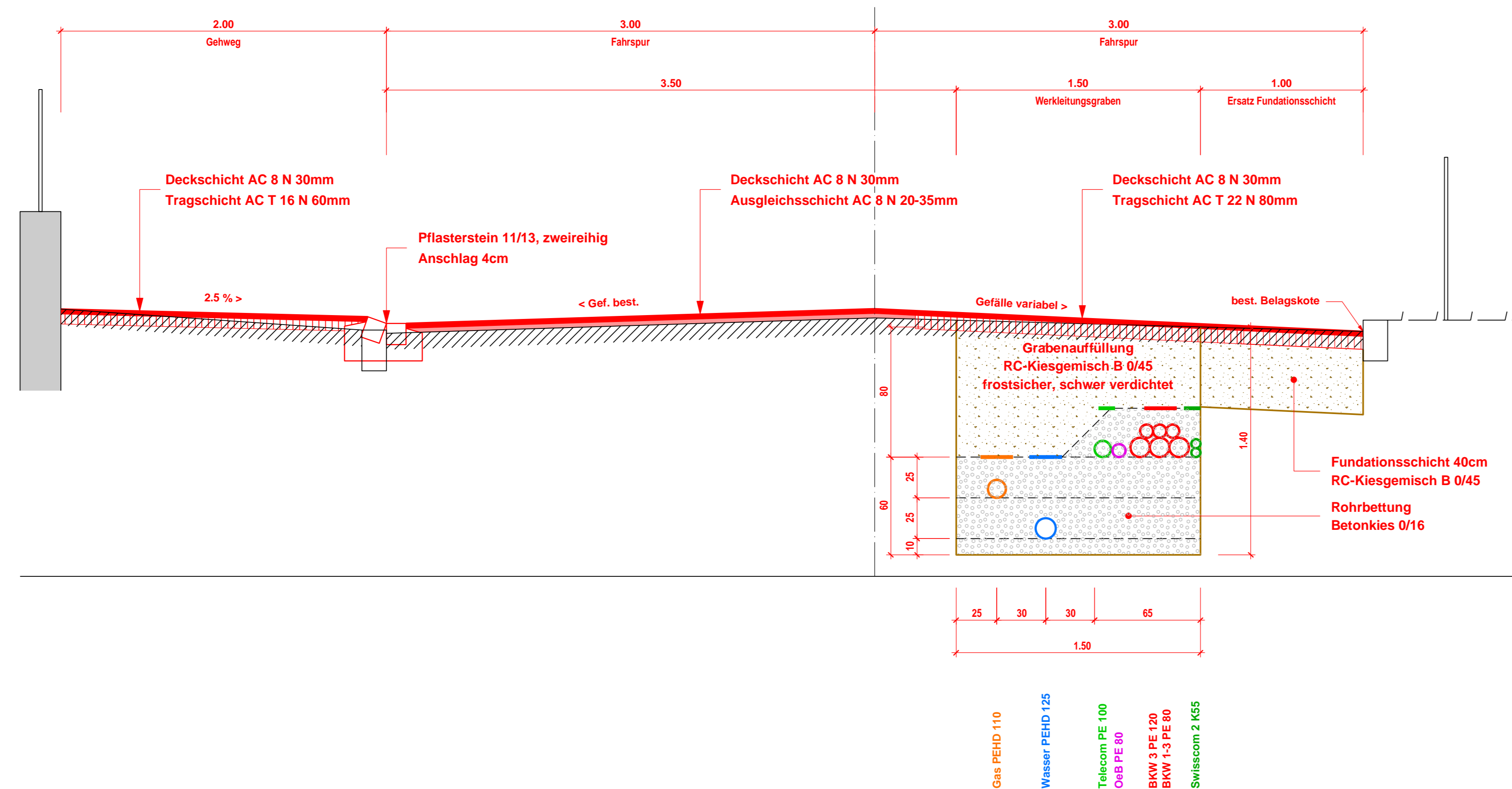
Normalprofil 2
