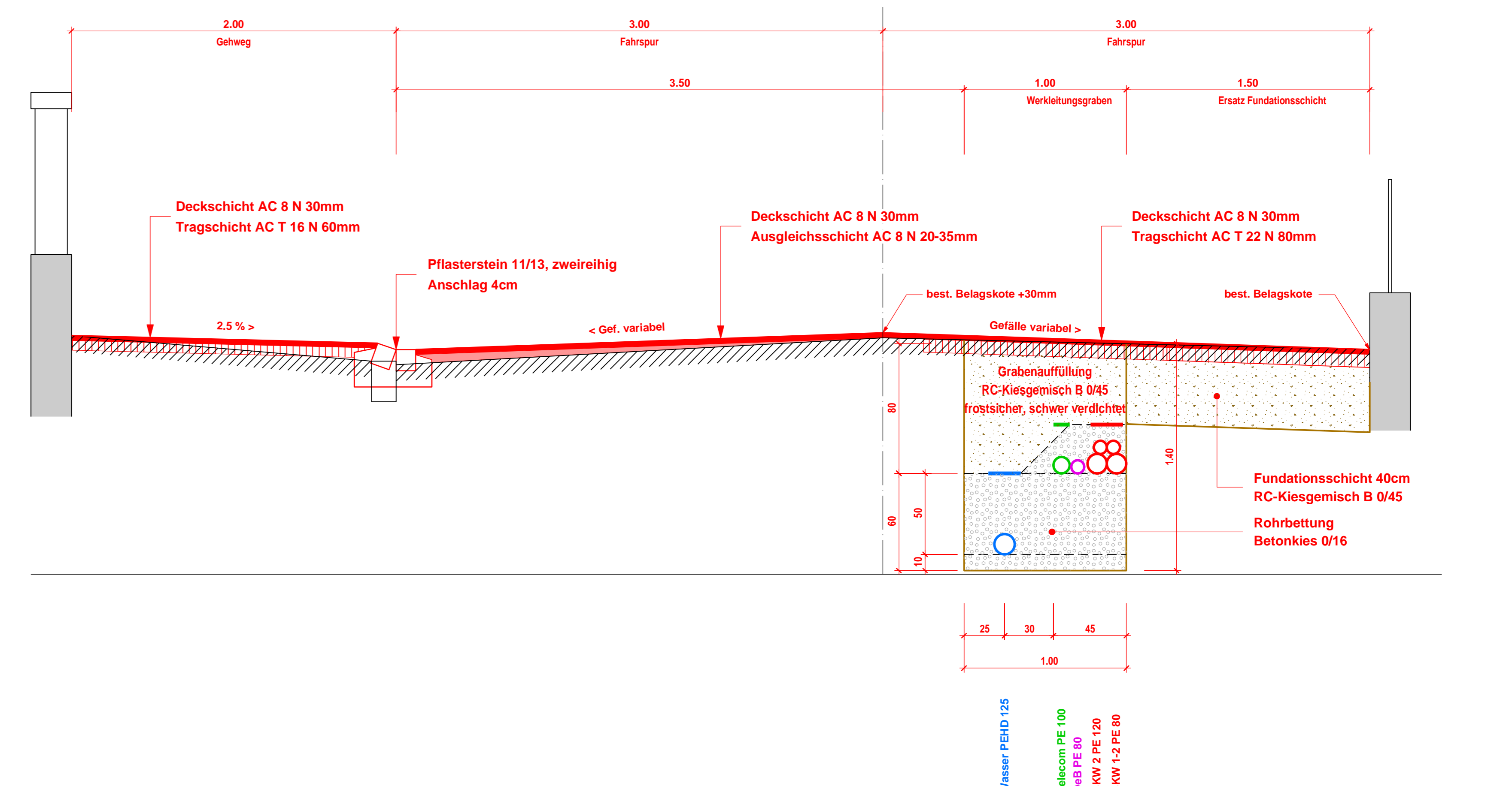
Normalprofil 4
