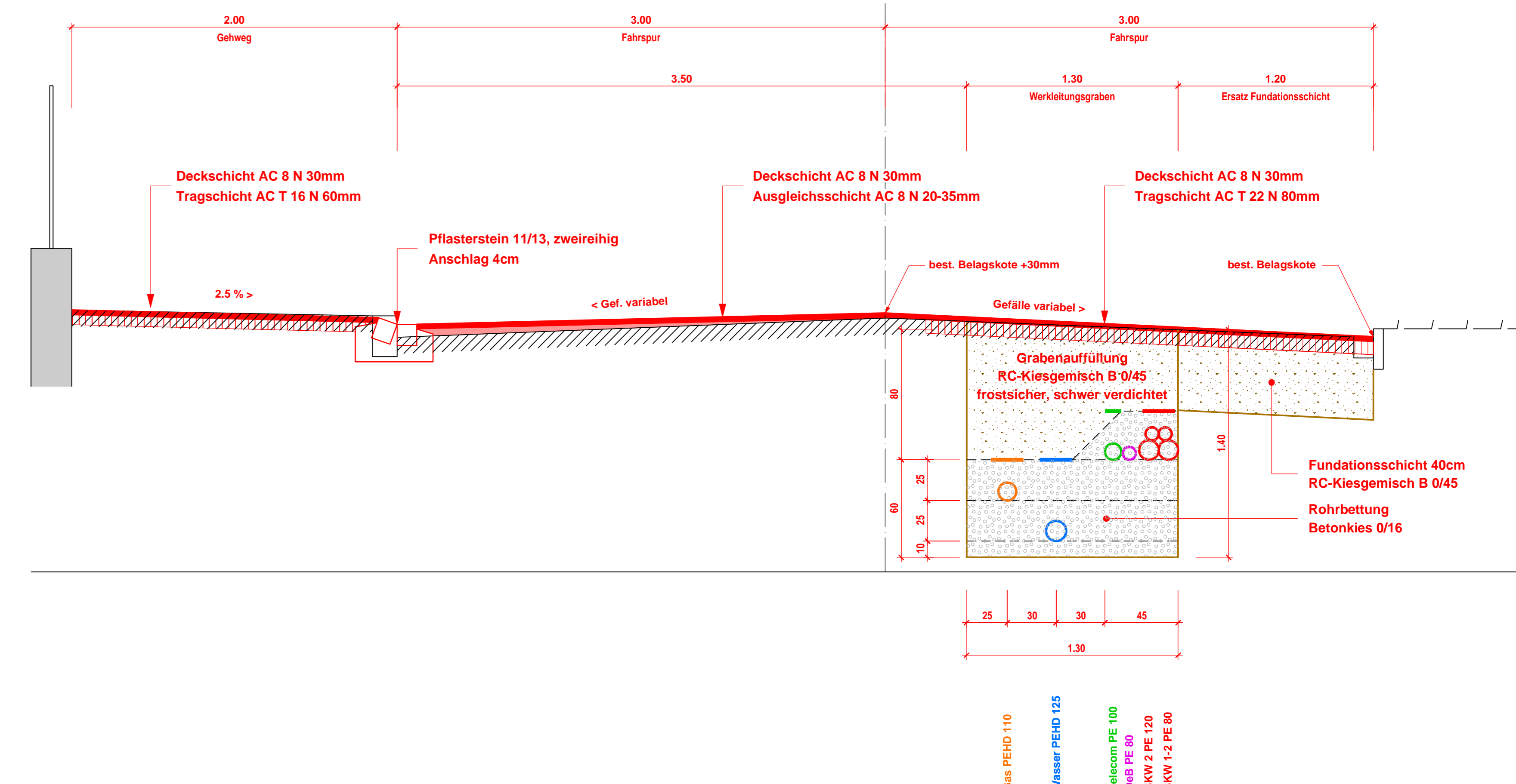
Normalprofil 3
